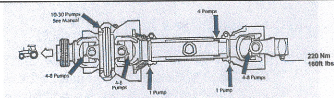
Fig.10 : Arbre d'entrée primaire
