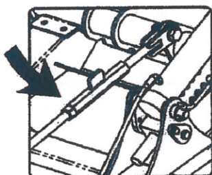
Fig.2 : Dispositif de réglage de l'horizontalité
